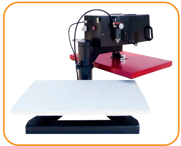
Fig. 3 - freistehender Druckteller
